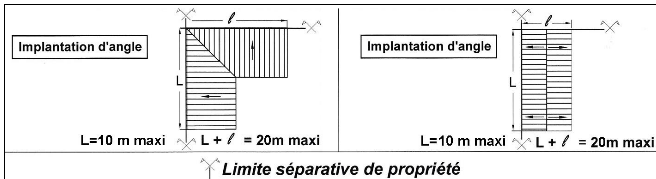
Façade sous sablière sur limites séparatives
